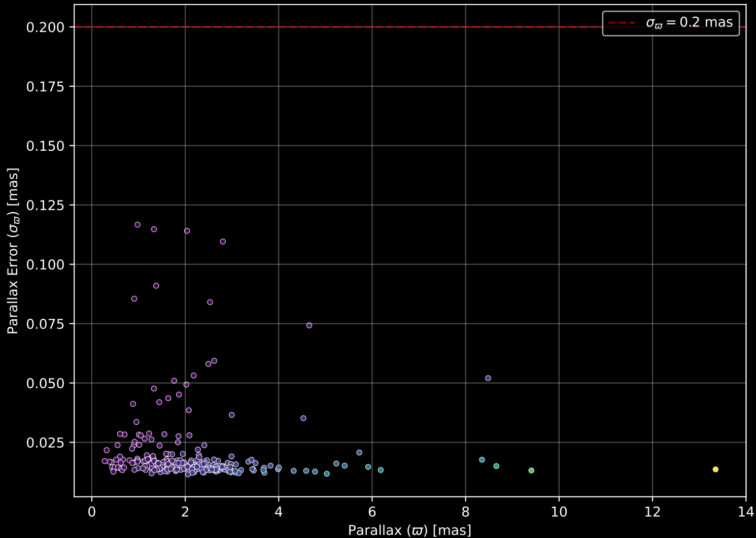
GALAH DR4 Field: [2562] Parallax Quality (n= 257)
