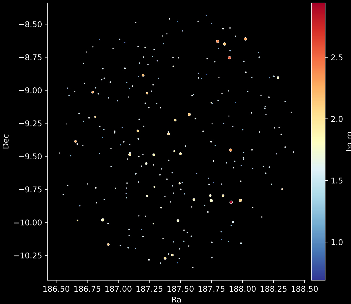
GALAH DR4 Field: [2562] Stars: 257
