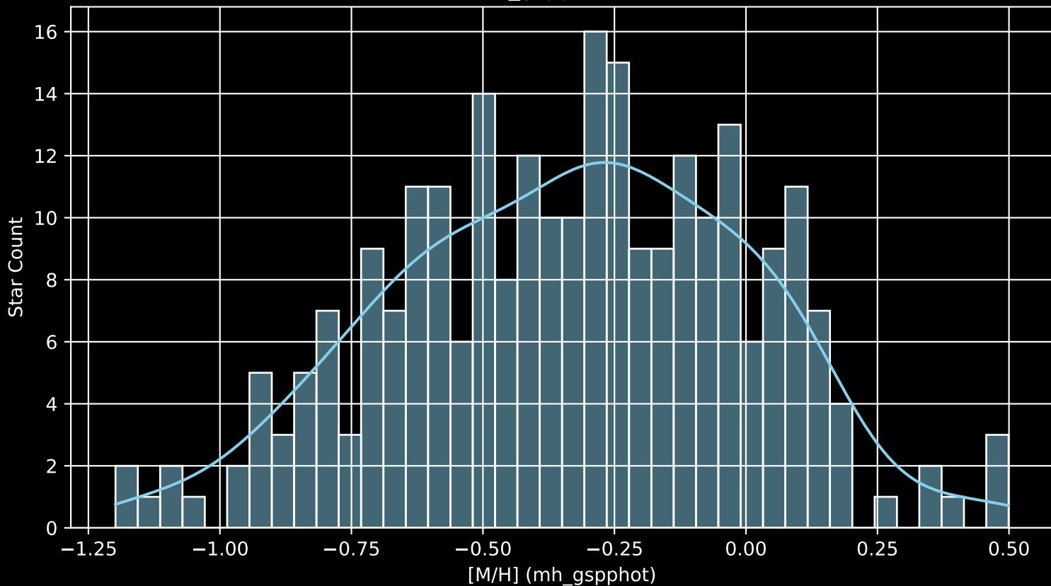
GALAH DR4 Field: [2562] [M/H] (mh_gspphot) (n= 257)
