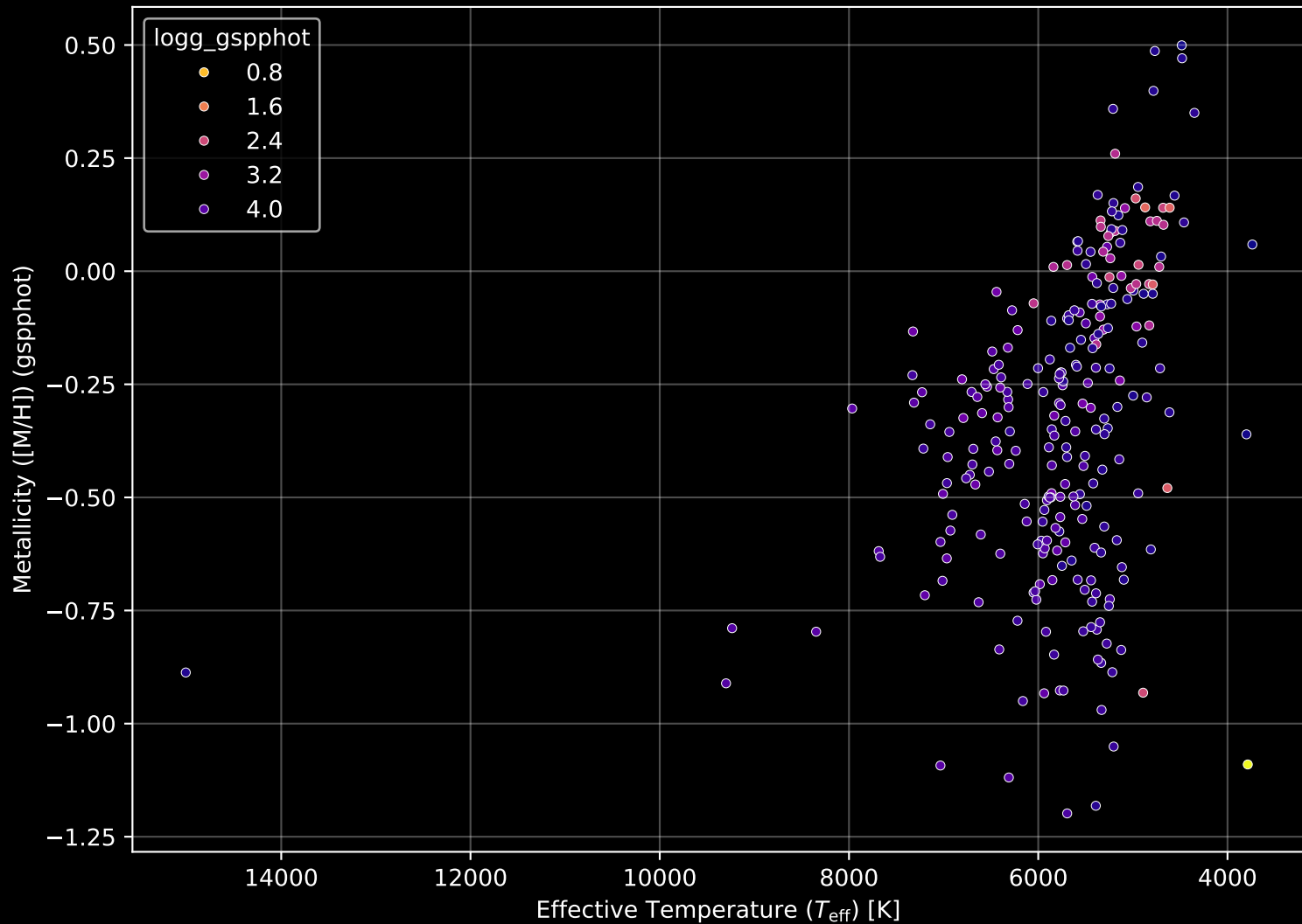
GALAH DR4 Field: [2562] Stellar Population Parameters (n= 257)
